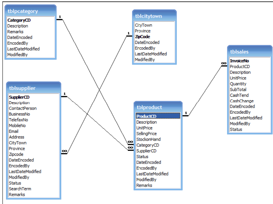
Gambar 5. Relasi Antar Tabel
