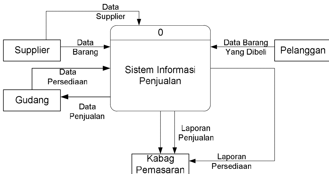
Gambar 3. Diagram Konteks pada Sistem Informasi Penjualan CV. Putra Mas Pratama Medan
