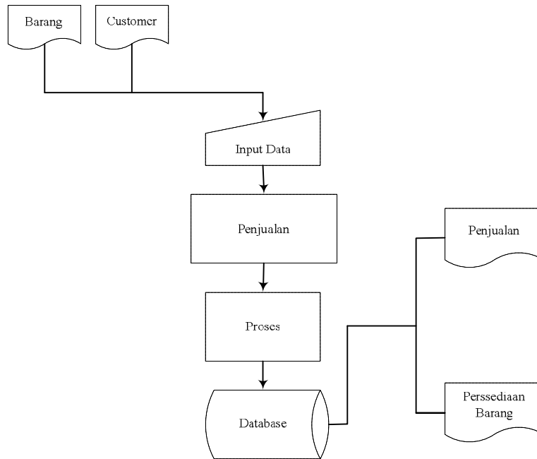
Gambar 2. Bagan Alir Sistem Informasi Penjualan Usulan
