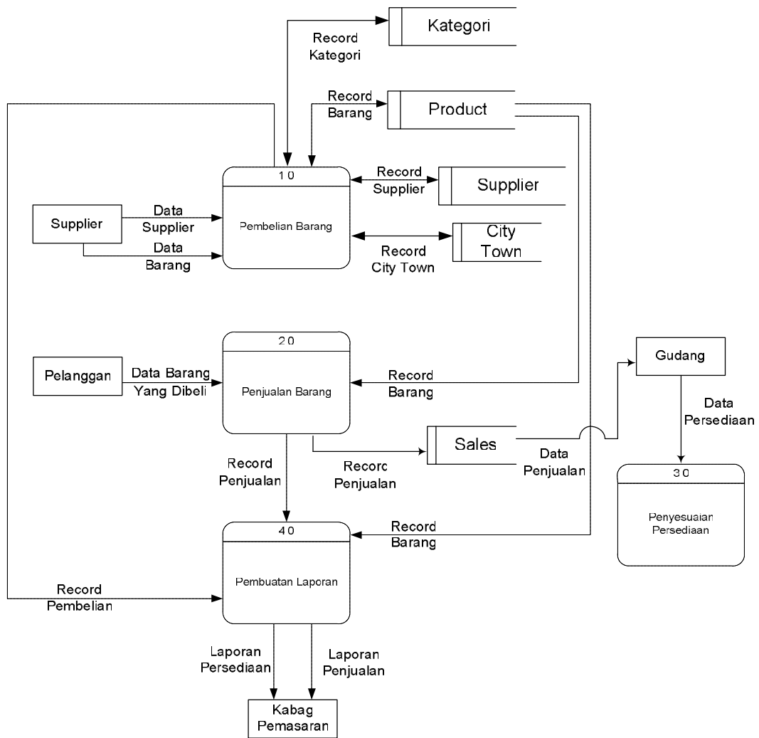
Gambar 4. DFD Level Nol Sistem Informasi Penjualan pada CV. Putra Mas Pratama Medan
